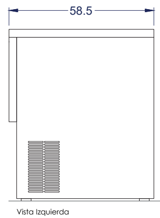
Vista Izquierda
