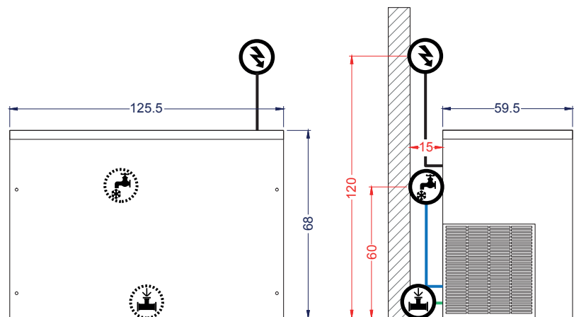
Vista Elevación
