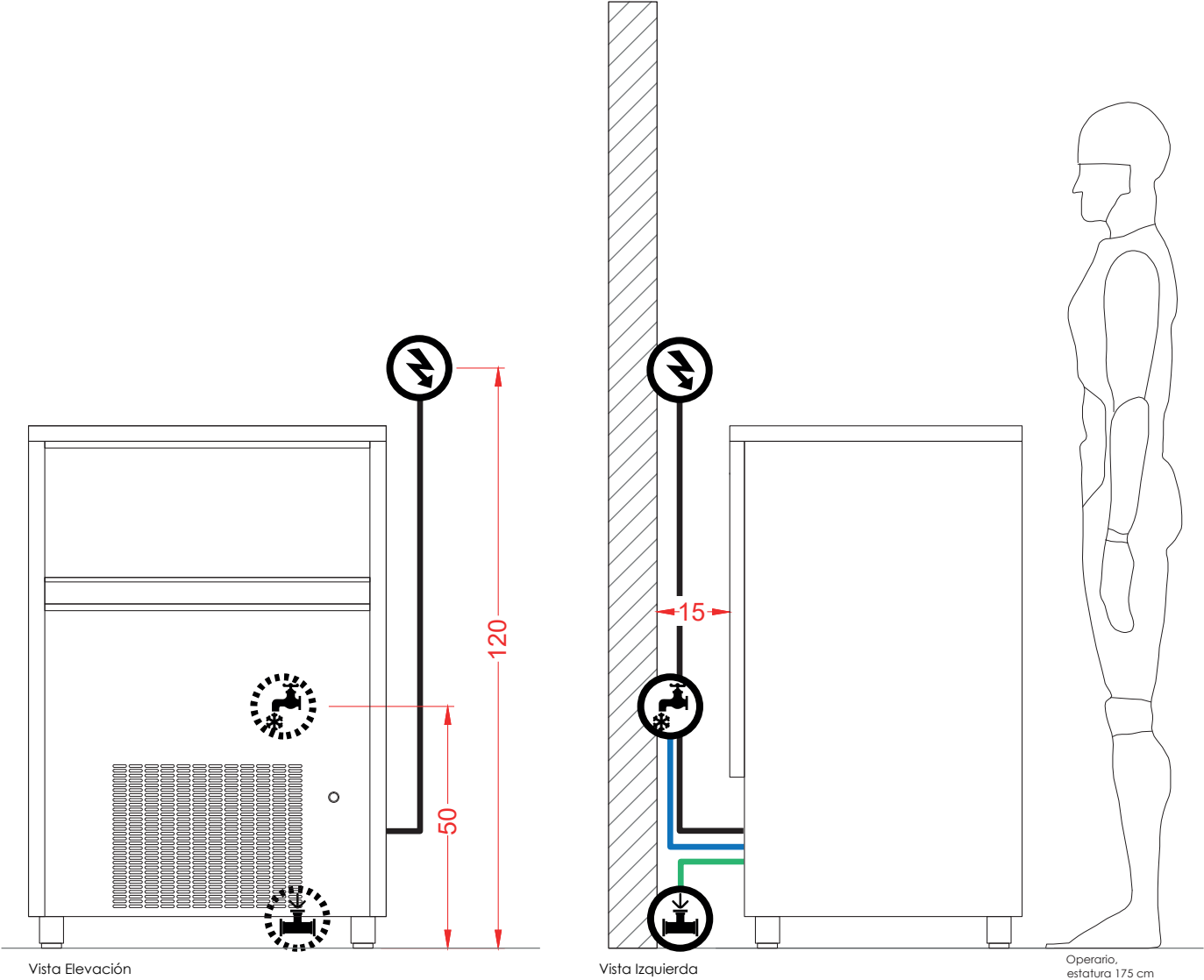
Vista Elevación
